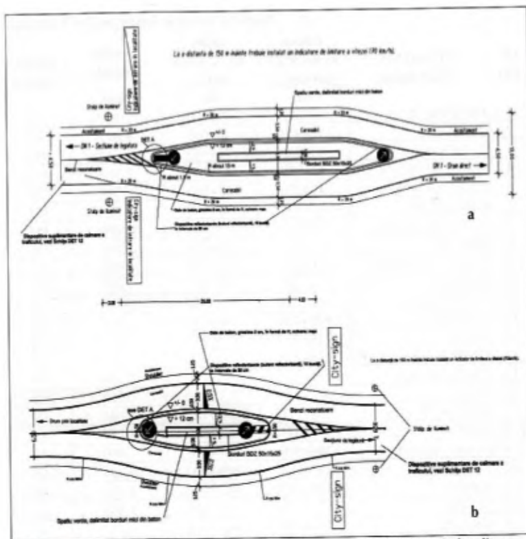
Calmarea traficului la intrarea în localitate - Insula de intrare în localitate
