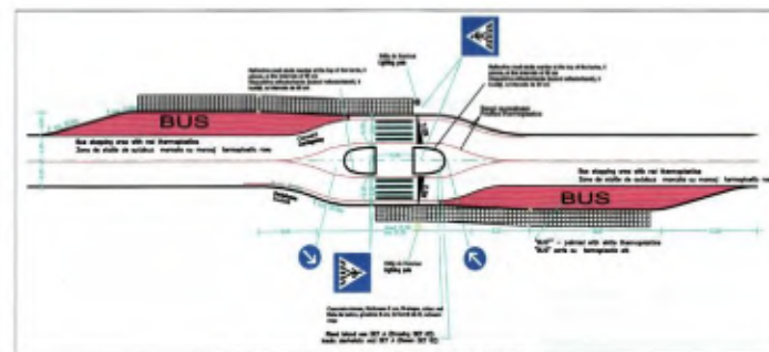
Trecere de pietoni combinată cu stații de autobuz
