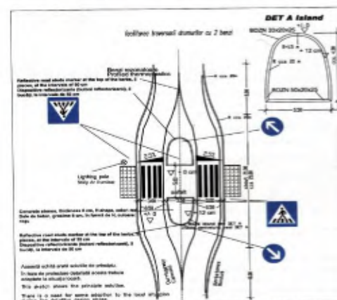
Insulă mediană pentru reglajul pietonilor - traversare în doi timpuri. Se aplică pe sectoarele cu două benzi de circulație
